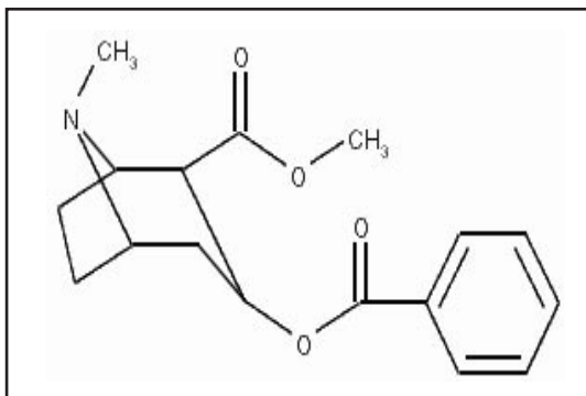
Figura 1. “Estructura de la cocaína”.
